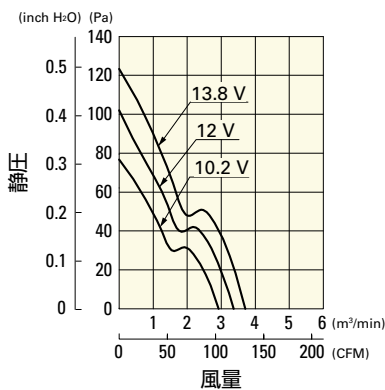
9WG1212E101-E パルスセンサ付
