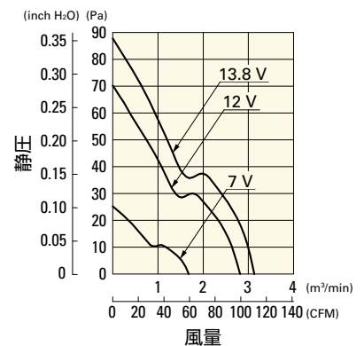
9WG1212H101-E パルスセンサ付
